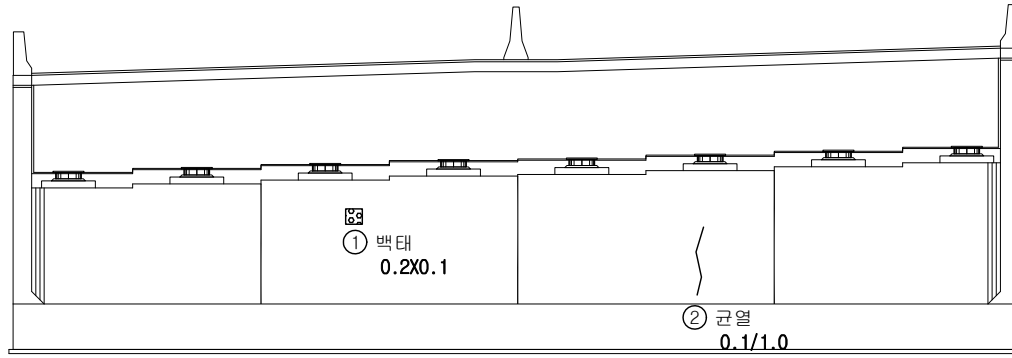
정면도
